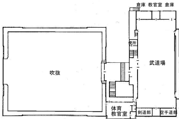
《2階平面図》
