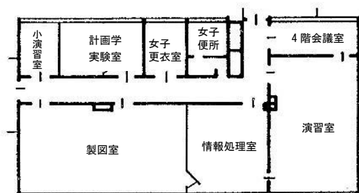
《4階平面図》
