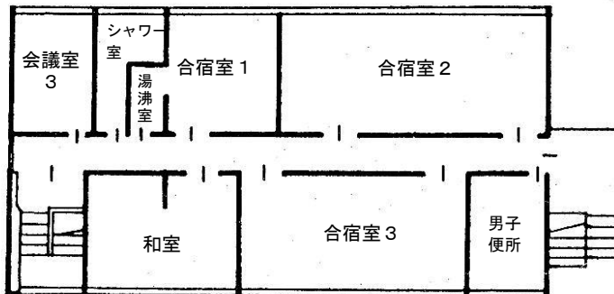
《3階平面図》
