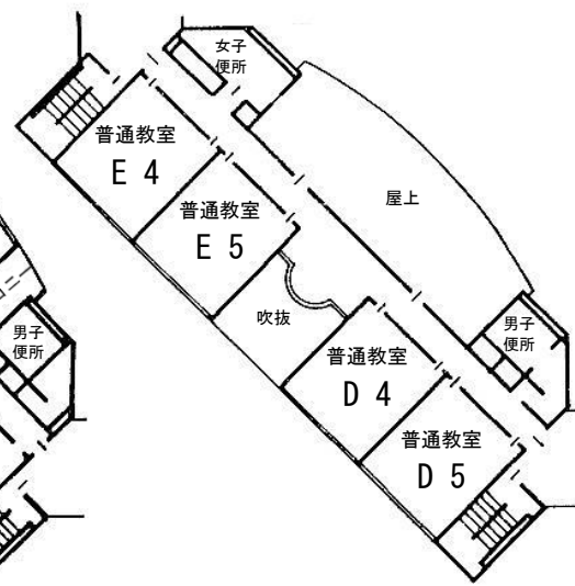
《4階平面図》
