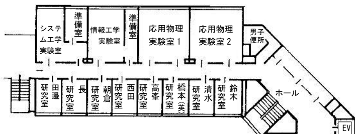
《2階平面図》
