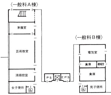
《1階平面図》
