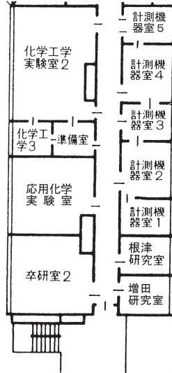
《2階平面図》
