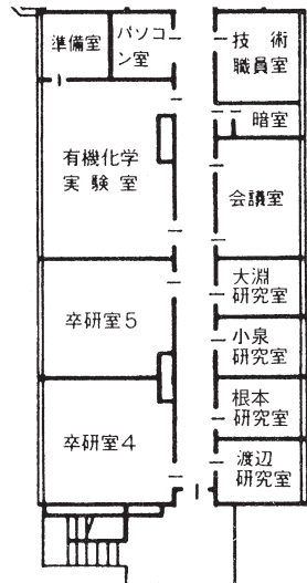
《4階平面図》
